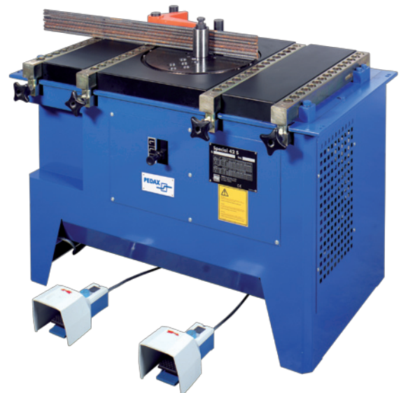
Special 42 S: Fast, powerful production machine for construction sites and bending shops, with robust pin control. // Special 42 S: máquina de producción rápida y potente para obras y talleres de curvado, con robusto mando de clavijas.
